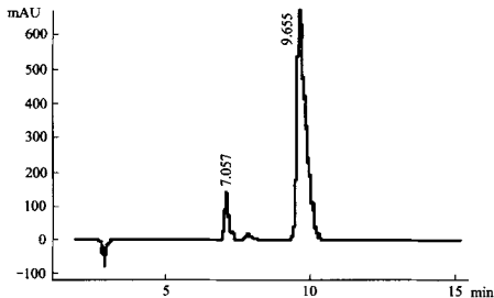
图 2 试样中喹禾灵 R、S 对映体拆分色谱图
